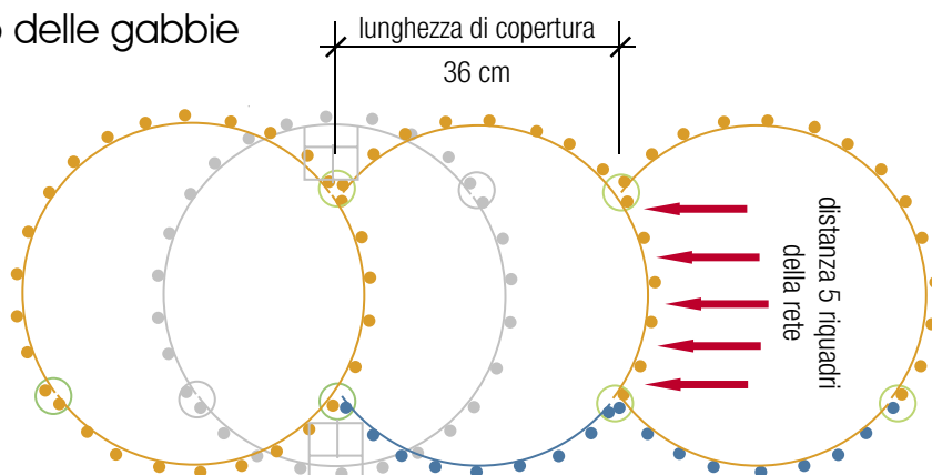
Montaggio delle gabbie d=52 cm
