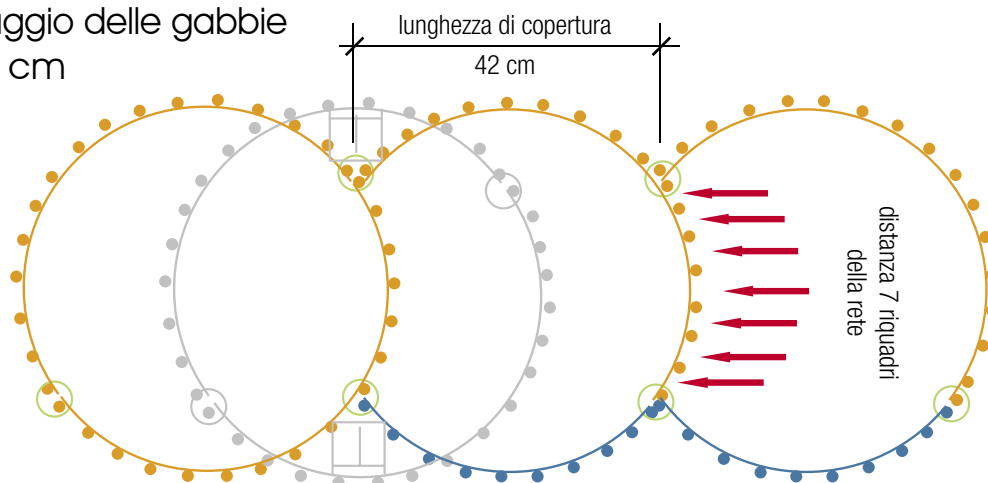
Montaggio delle gabbie d=65 cm
